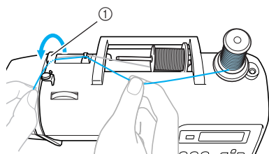
① Couverture du guide-fil
