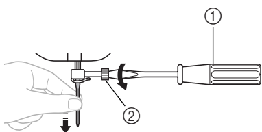
① Screwdriver / Destornillador ② Needle clamp screw / Tornillo de la presilla de la aguja
