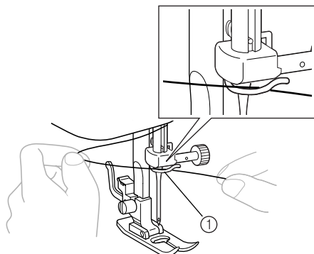
① Needle bar thread guide / Guía del hilo de la varilla de la aguja
