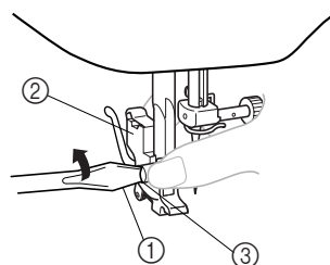
① Screwdriver / Destornillador ② Presser foot holder / Soporte del pie prensatela ③ Presser foot screw / Tornillo del pie prensatela
