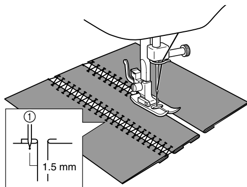
① First needle drop / Primera entrada de la aguja
